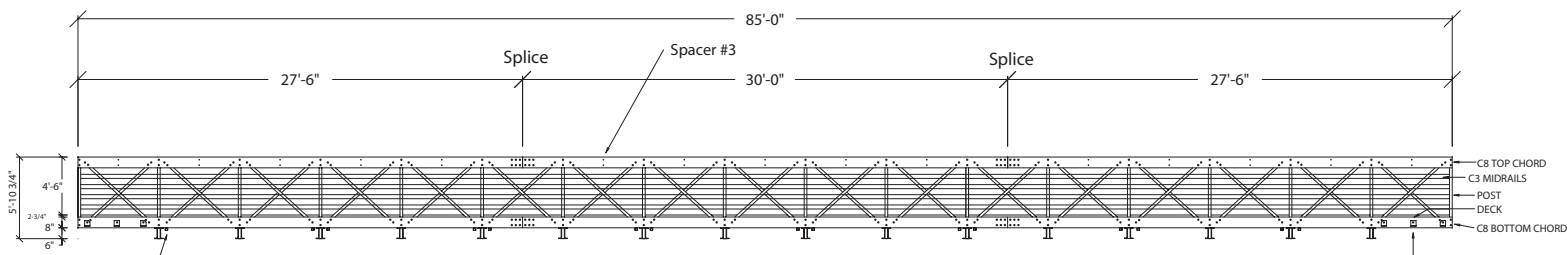
ELEVATION
